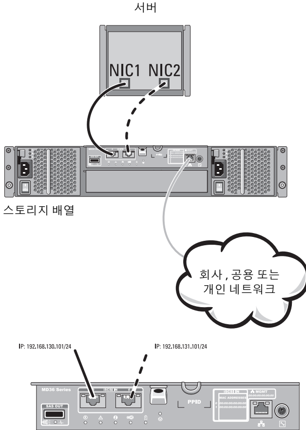
그림 2-2. 단일 컨트롤러에 연결된 1 개의 호스트
