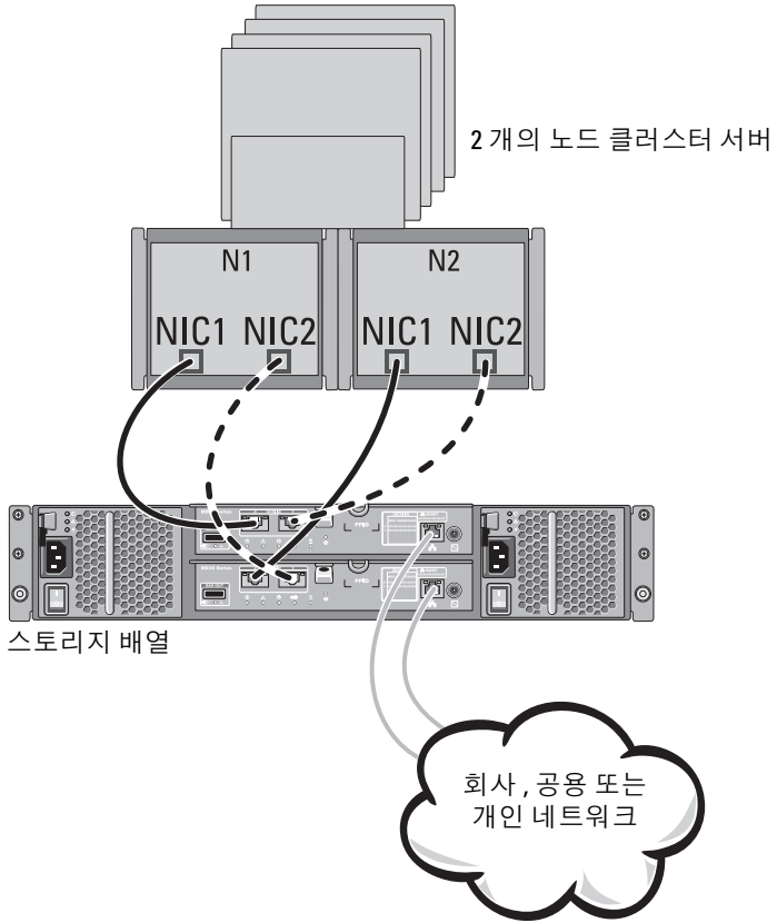
그림 2-5. 이중 컨트롤러 구성에 연결된 2 개의 호스트
