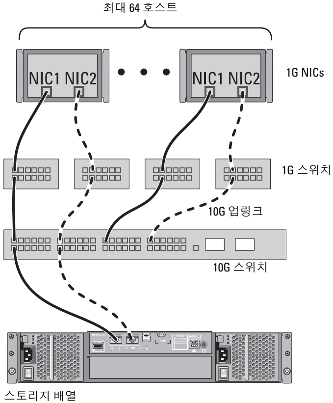
그림 2-8. 단일 RAID 컨트롤러에 연결된 64 개의 서버
