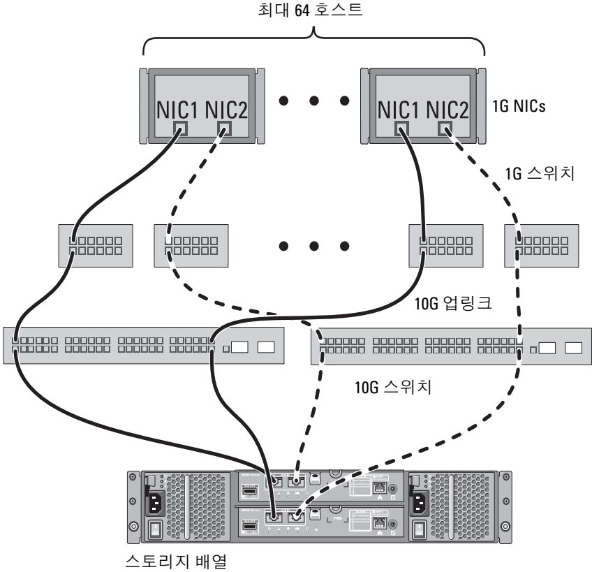
그림 2-9. 2 개의 RAID 컨트롤러에 연결된 64 개의 서버
