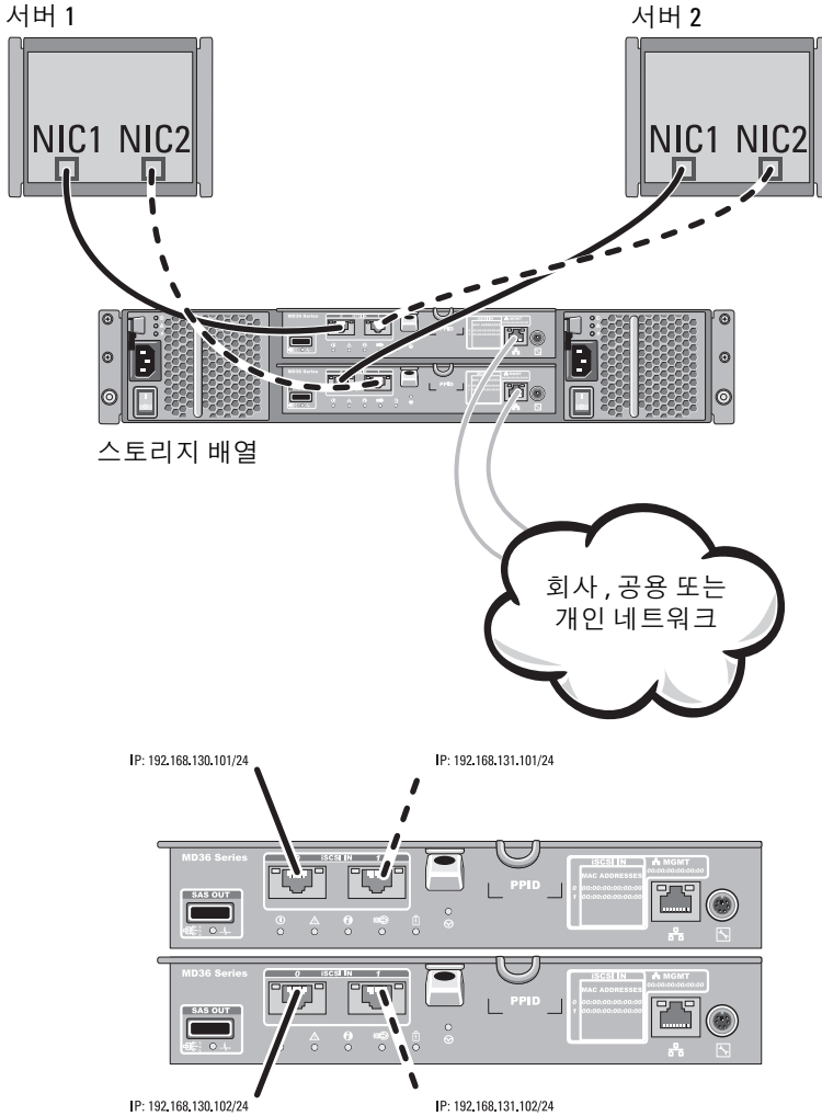
그림 2-4. 2 개의 컨트롤러에 연결된 2 개의 호스트
