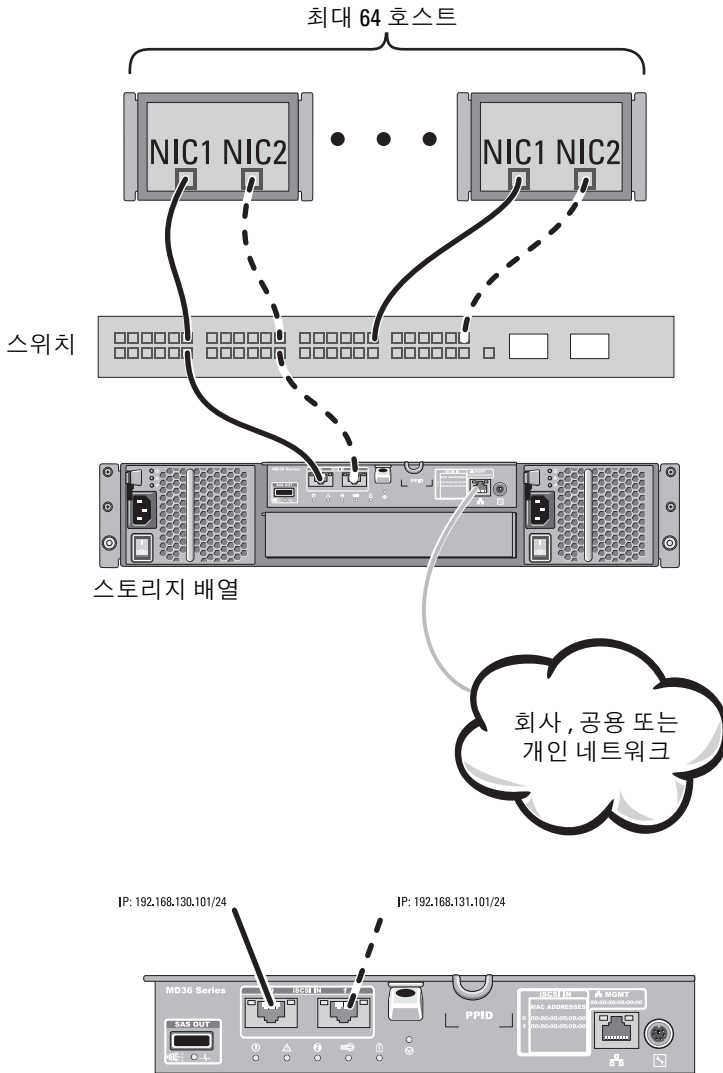
그림 2-6. 단일 컨트롤러에 연결된 64 개의 서버
