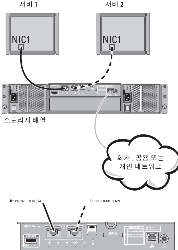
그림 2-1. 단일 컨트롤러에 연결된 2 개의 호스트
