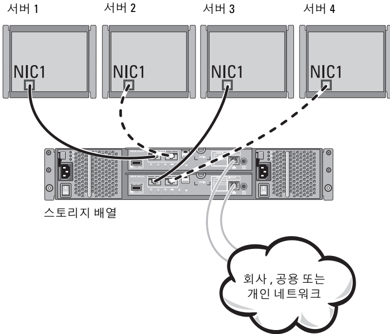
그림 2-3. 이중 컨트롤러 구성의 4 개의 호스트
