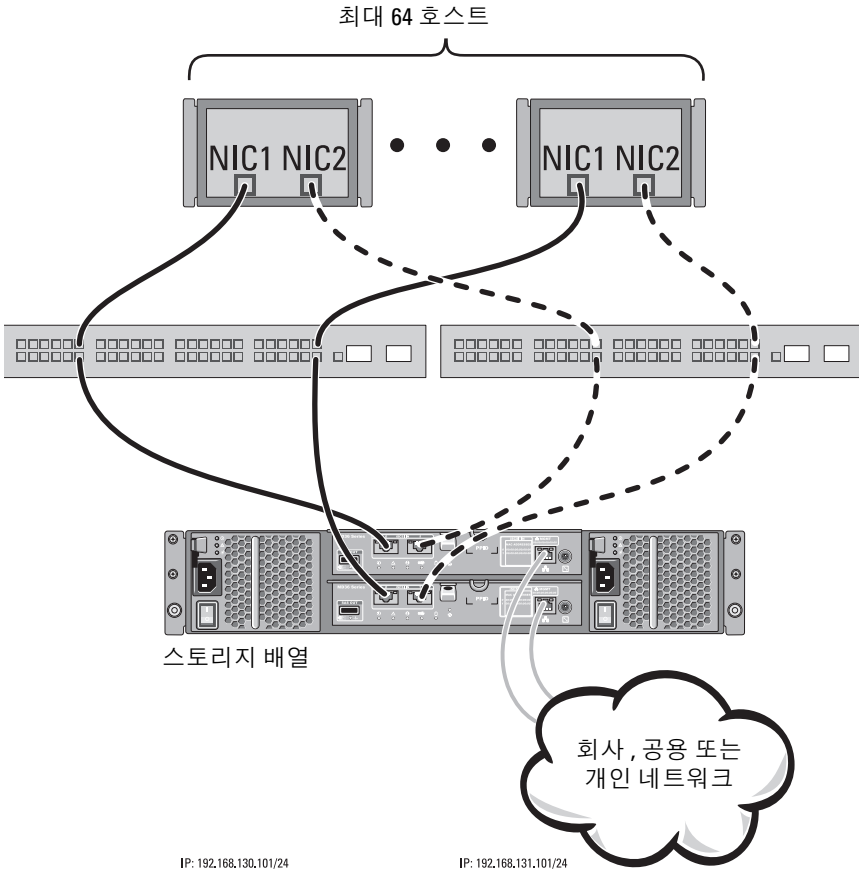
그림 2-7. 2 개의 컨트롤러에 연결된 64 개의 서버
